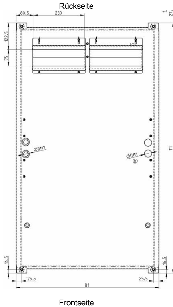
Abmessungen Deckel mit Kabeleingängen 12- 17 - 25 / 35 kW (Draufsicht)
